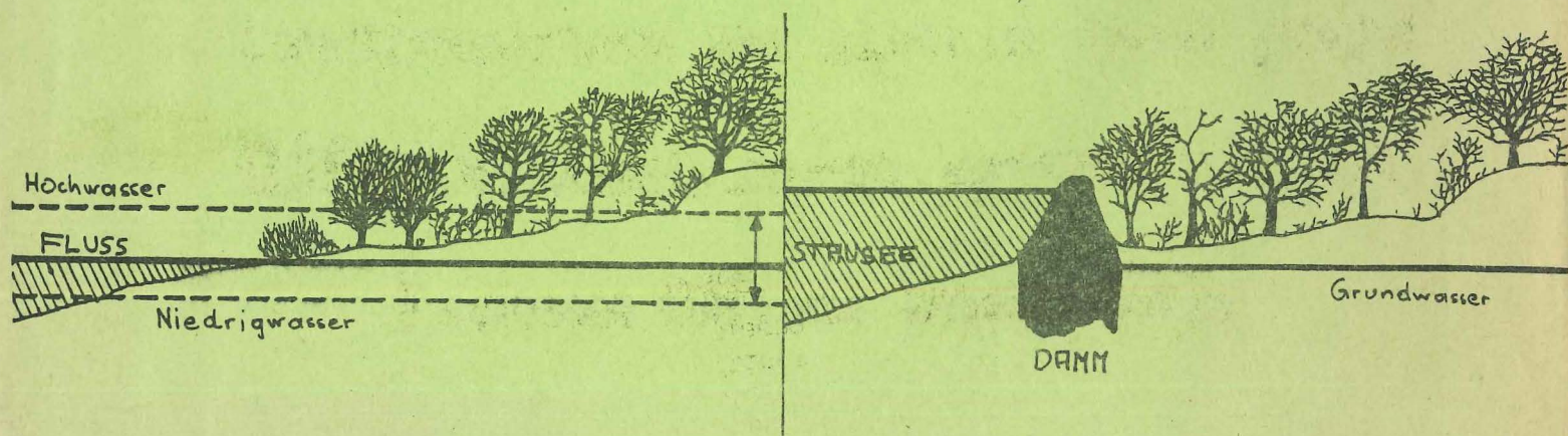
Querschnitt des Flußufers (nicht maßstabsgetreu)
