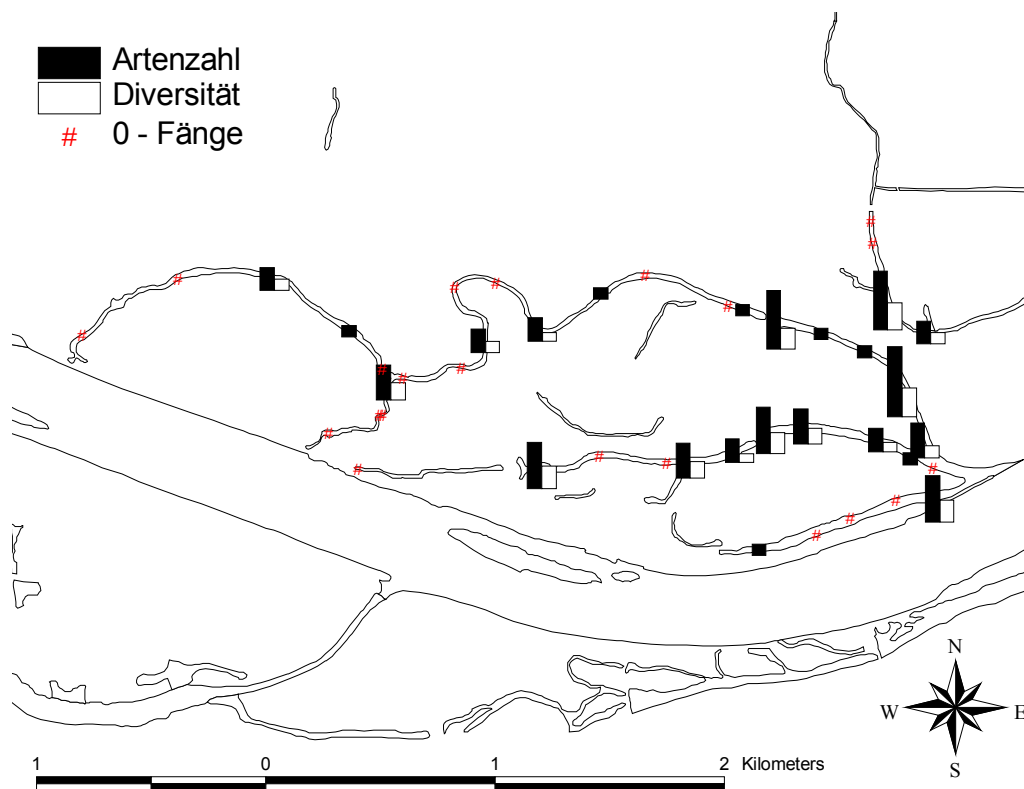
Abb. 4: Mollusken: Artenzahlen und Diversitäten im Untersuchungsgebiet.
